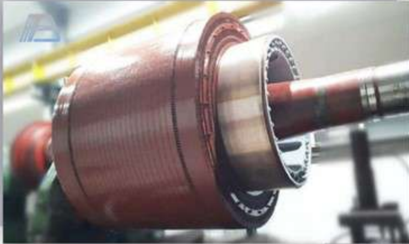
Капитальный ремонт якоря П22/145-4,56 (ПБК 250/145) 3600 кВт. Вес якоря 50 тн.
